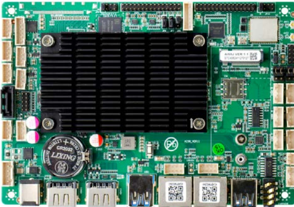
AI58J VER:1.1 主板正面图
