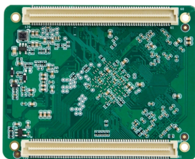
CK33H VER:1.2 主板背面图
